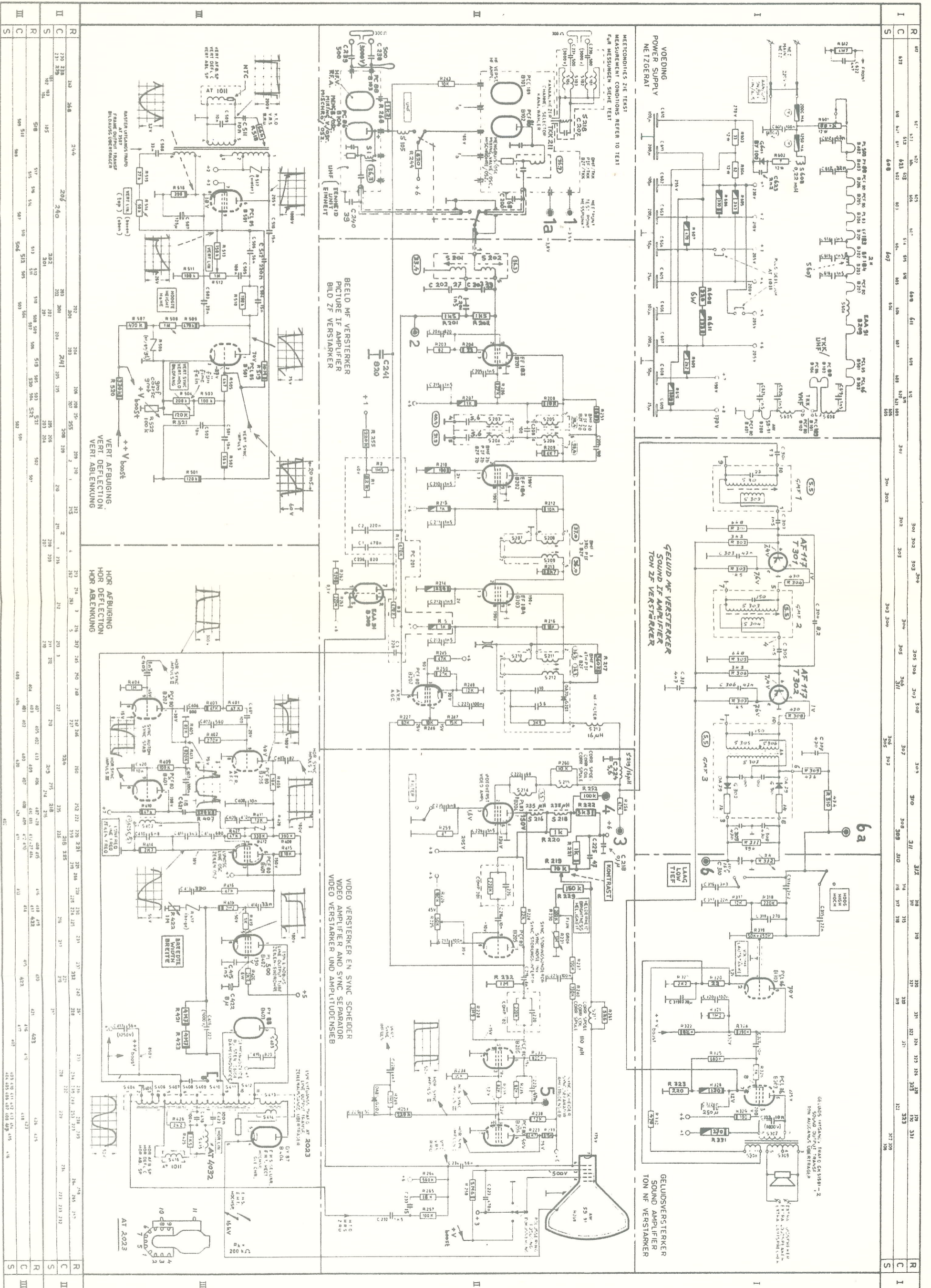
PRINCIPLE SCHEMA SCHEMATIC DIAGRAM PRINZIPSCHALTBILD TV 5637 T - TV 5637 T UHF
